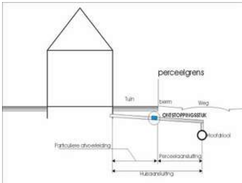
Figuur. Aansluiting op vrijvervalriolering
